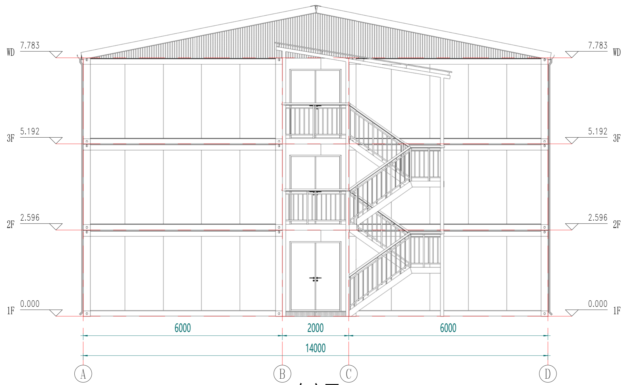
东立面
