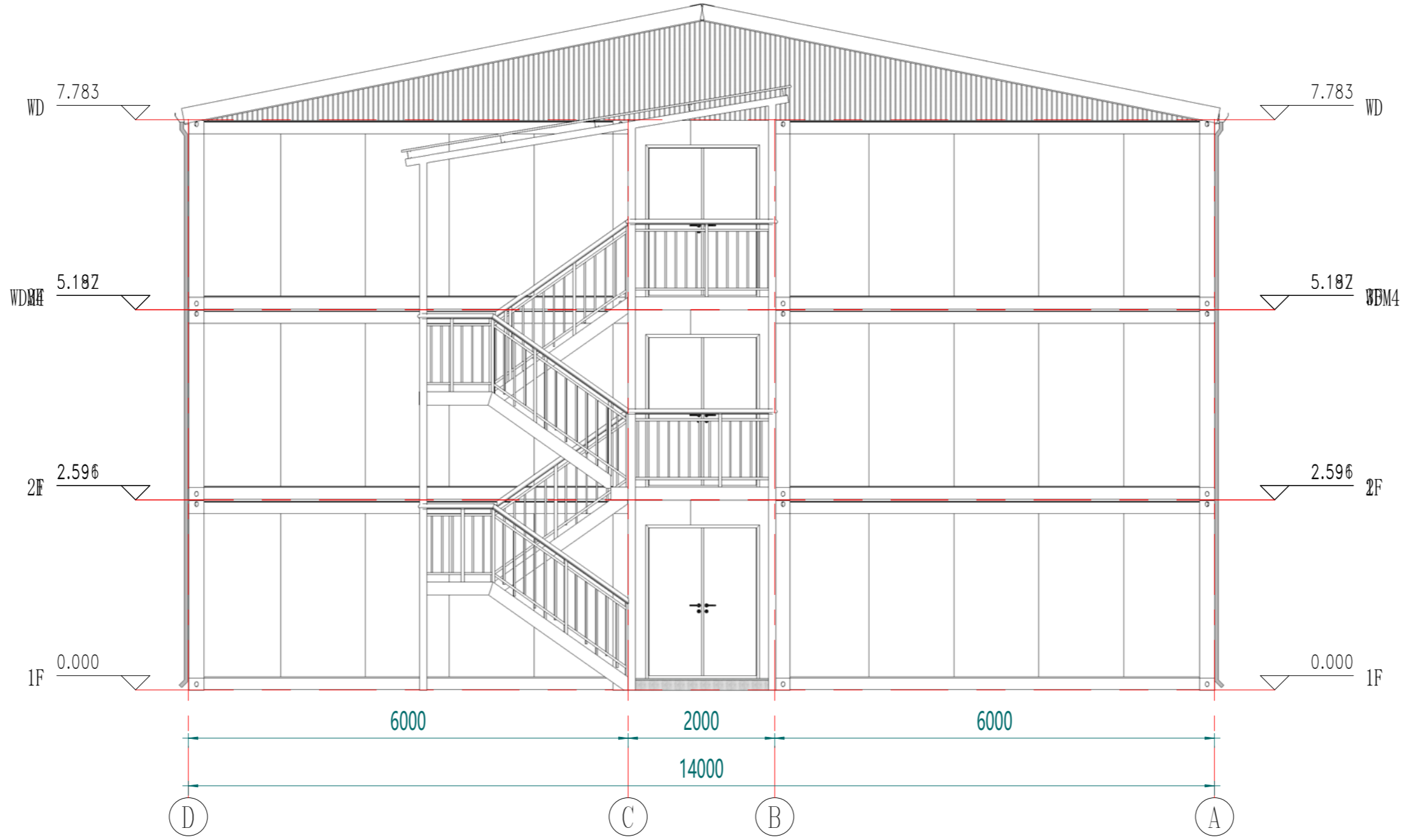
西立面
