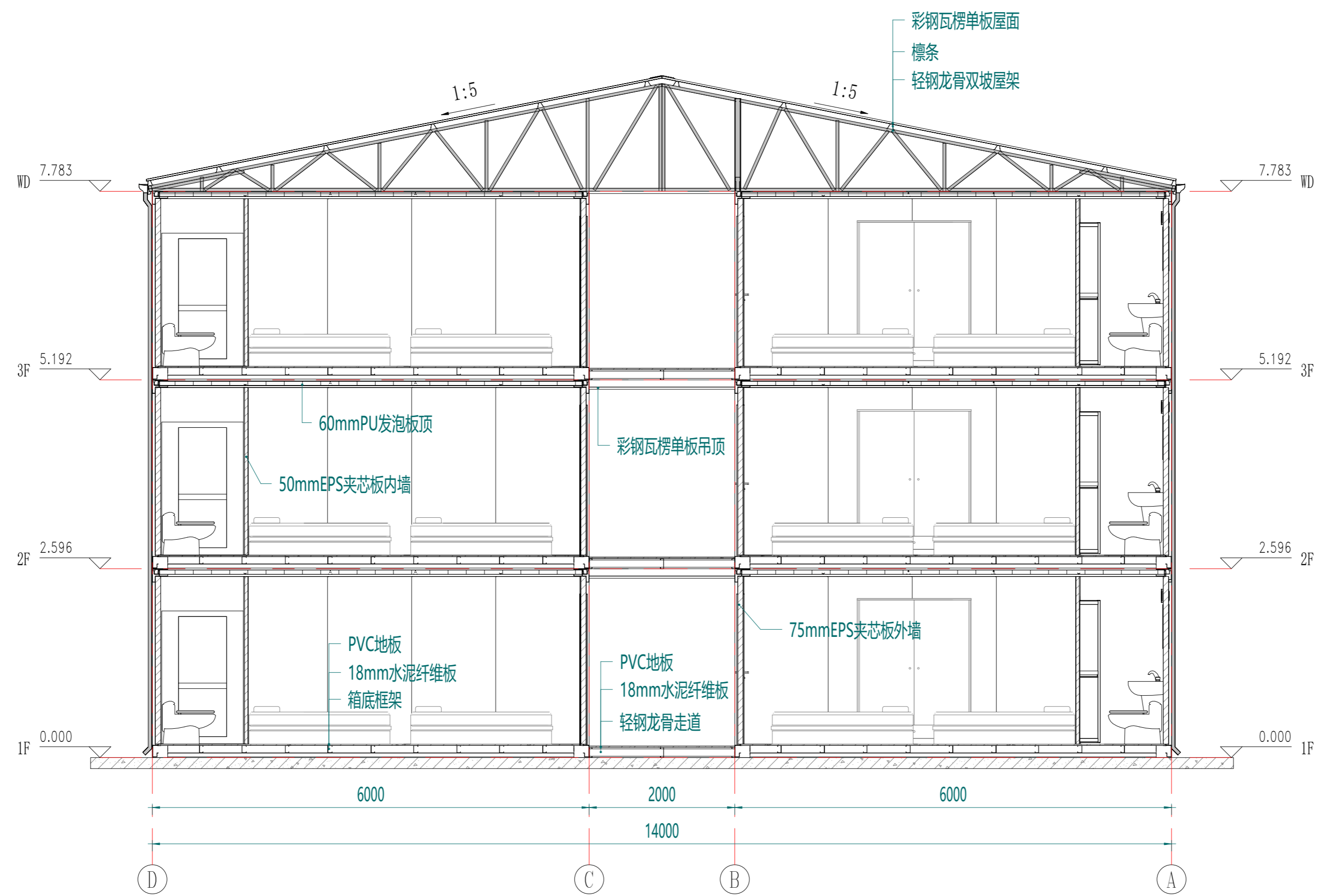
剖面布置图
