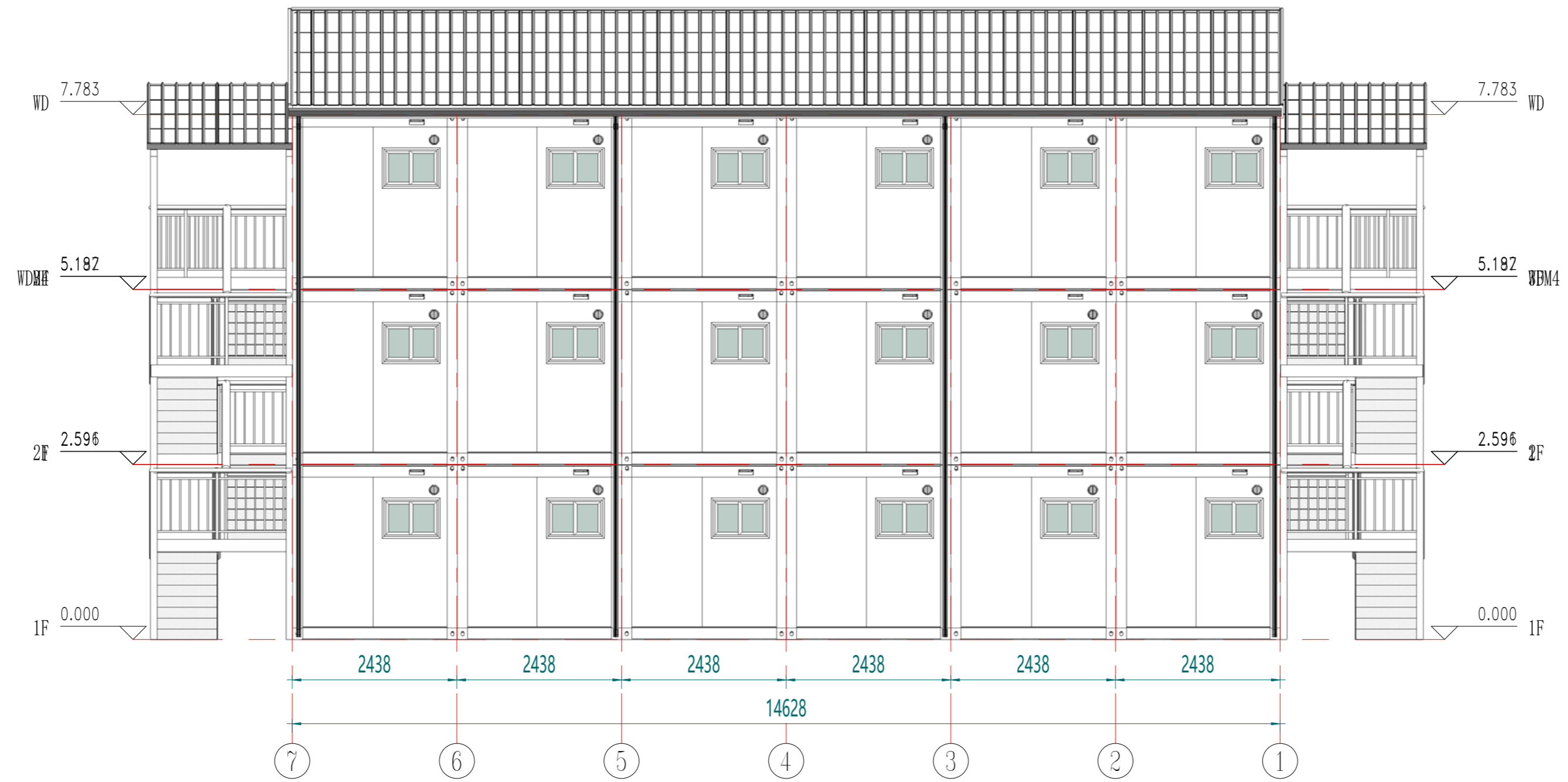
北立面
