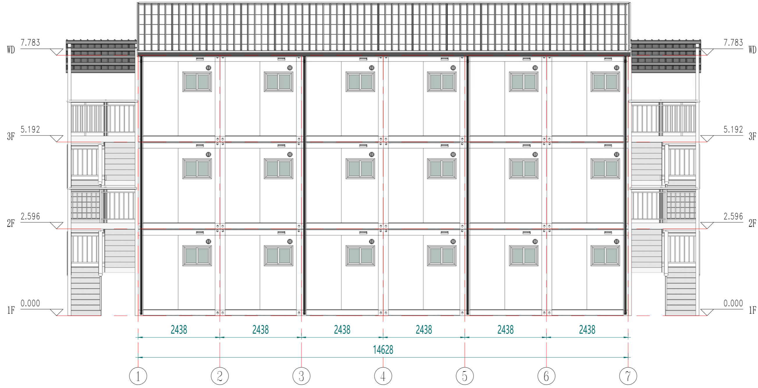
南立面
