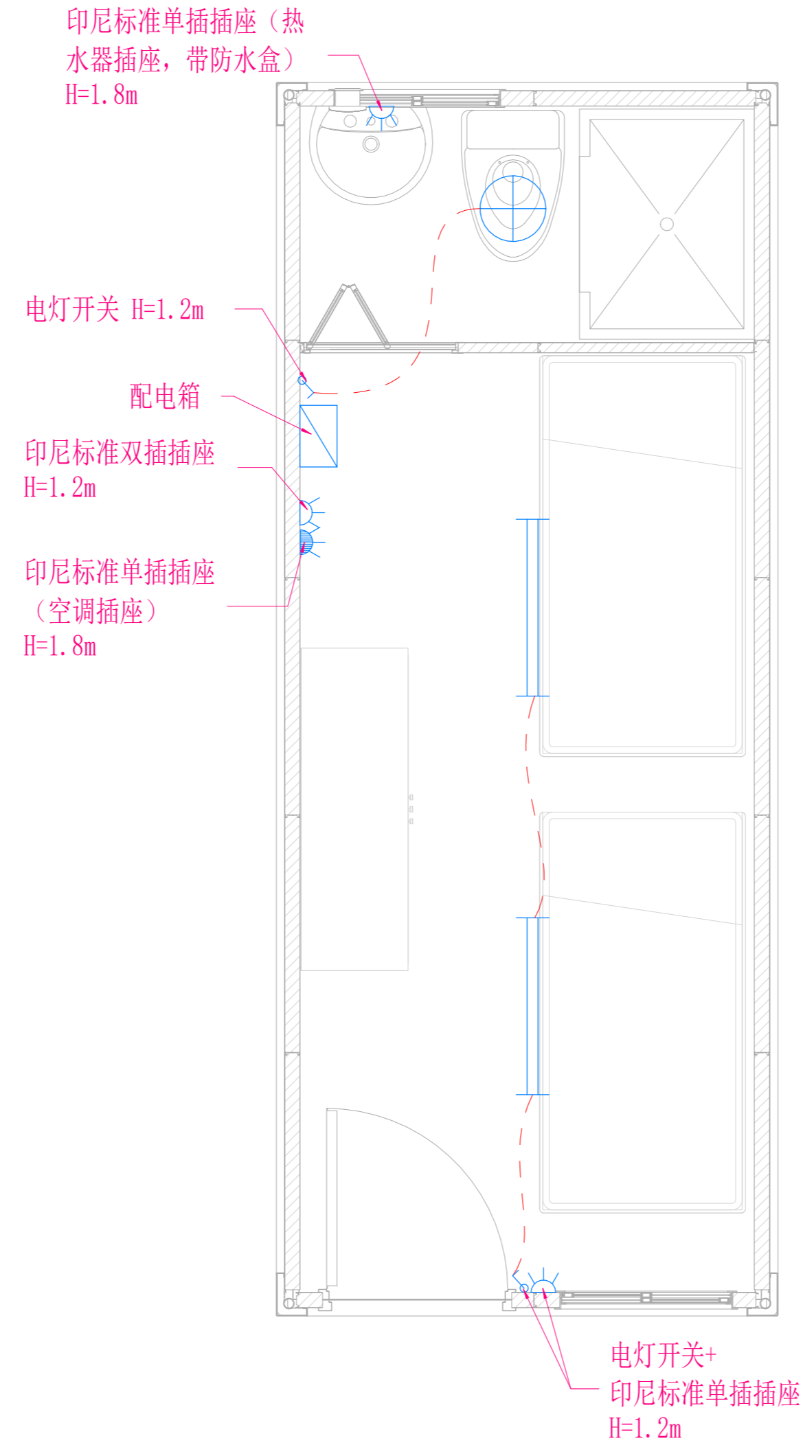
标准间电力布置图
