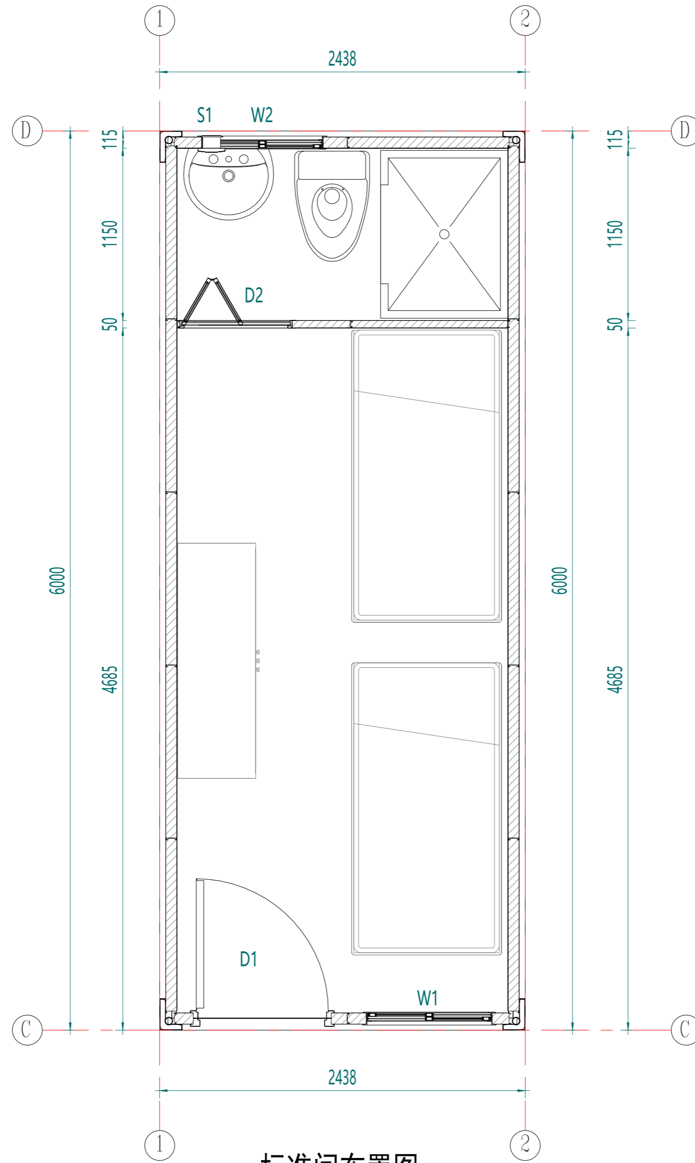
标准间布置图
